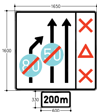
Σχήμα 3: Πινακίδες καθοδήγησης σε περιοχές πρόσθετης λωρίδας σε τμήματα ανωφέρειας
